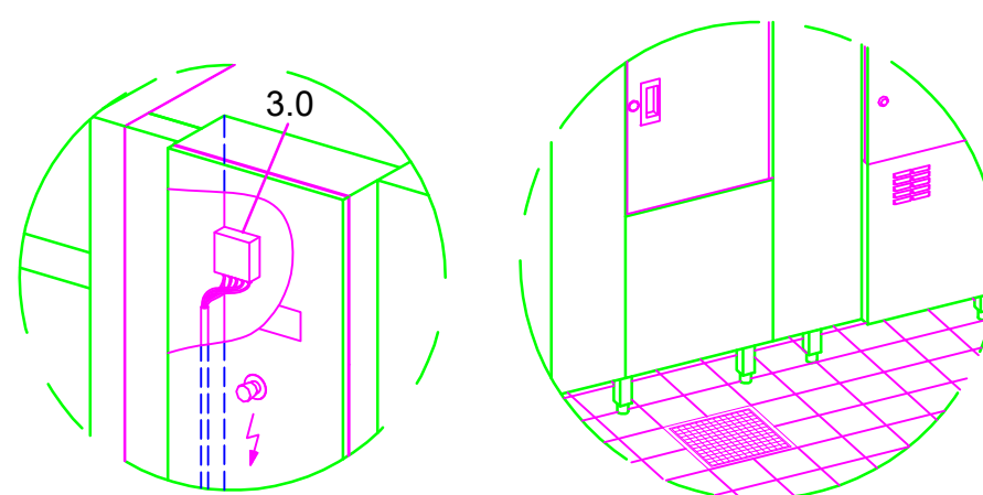
Przyłącza elektryczne w szafie sterowniczej zmywarki
